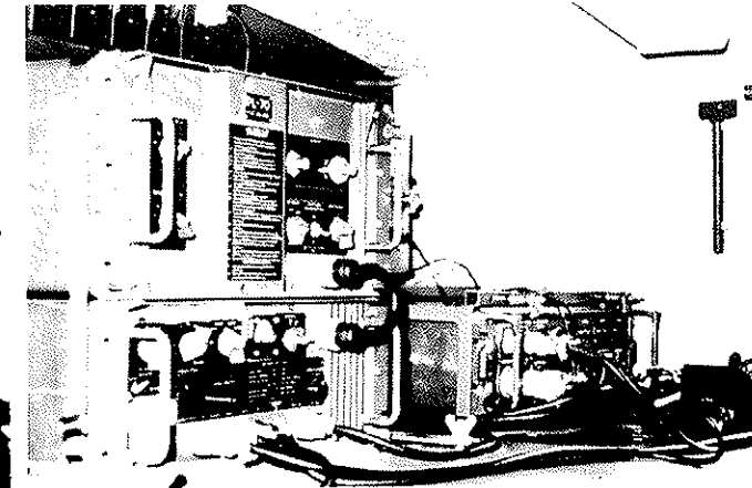
Panssariprikaatin liikkuvuudesta johtuen tulee viestiasemien olla asennettuina ajoneuvoihin. Tässä sisäkuva AS PL-70-linkkiausasta.
