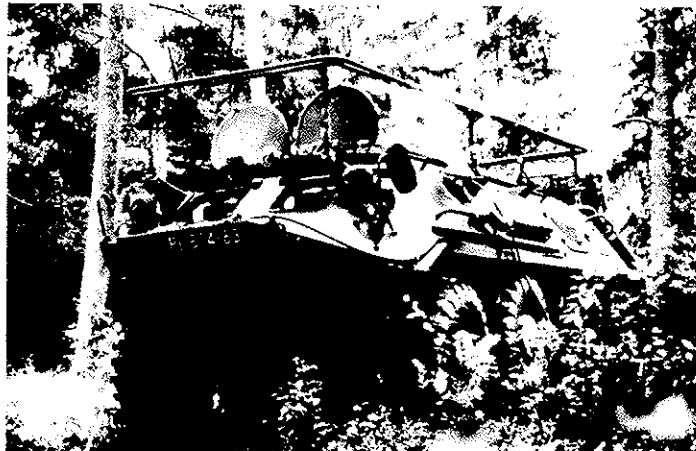
PsVK:n koulutuskaluston vaativinta ja uusinta linjaa edustaa esikuntapanssarivaunu BTR 60 PU. Kuvassa asema toimintakunnossa. Antennina VHF:lle laajakaista-antenni 16 metrin teleskooppimastossa sekä putkiantenni HF-alueelle.
